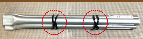
■管材まとめ (1本あたり耐荷重 AK8の場合15kg)
